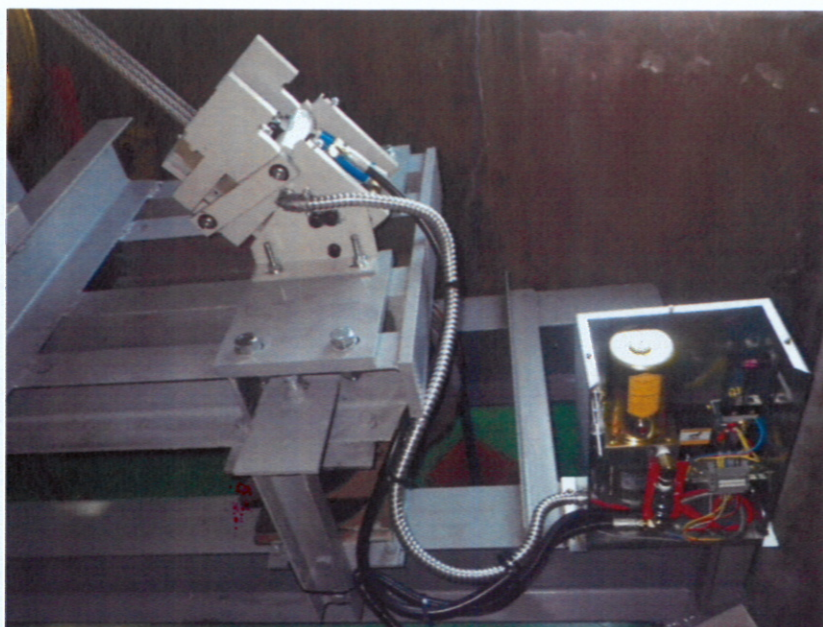
東棟 施工後 ロープブレー キ③
