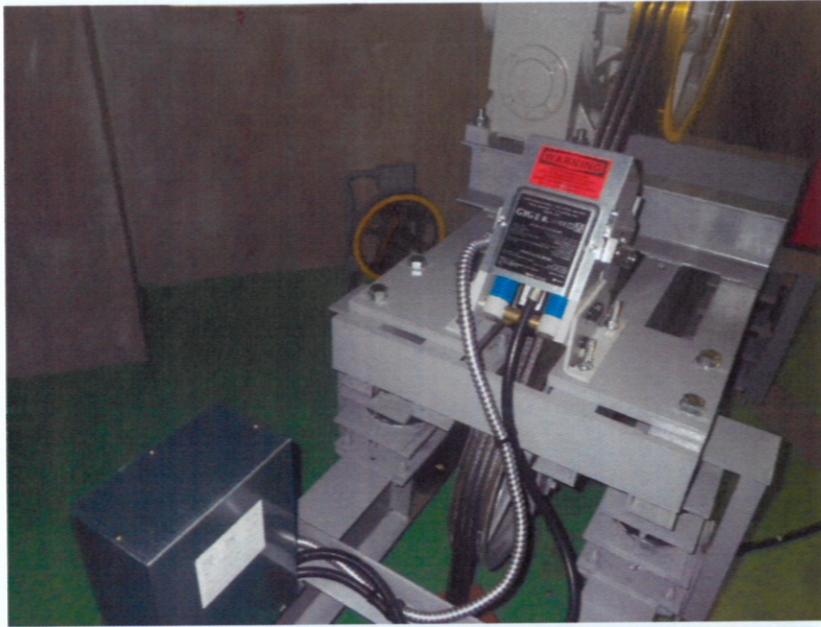
西棟 施工後 ロープブレー キ②
