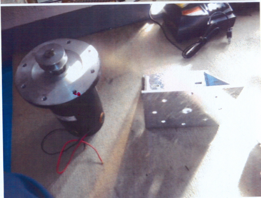
西棟 施工中 かご上ドアモ ーター
