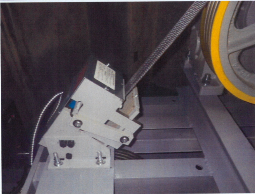
西棟 施工後 ロープブレー キ③
