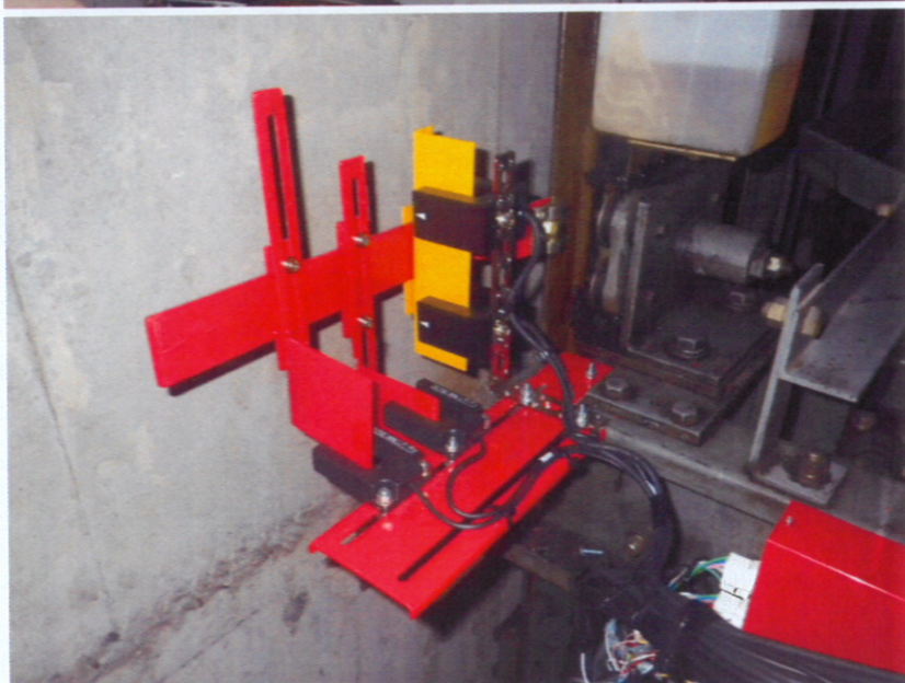
西棟 施工中 かご上近接ス イッチ③
