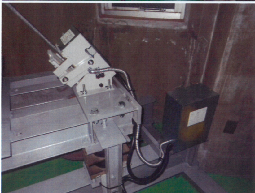
東棟 施工後 ロープブレー キ④
