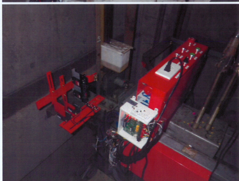
東棟 施工後 かご上ジャン クションボッ クス②
