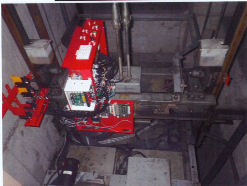
西棟 施工中 かご上近接ス イッチ②
