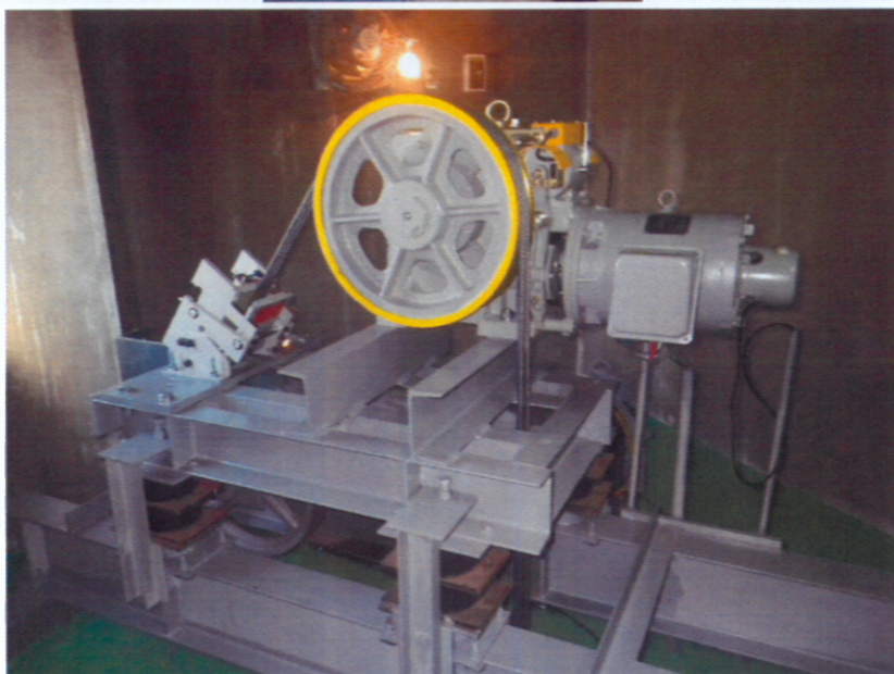
東棟 施工後 巻上機①
